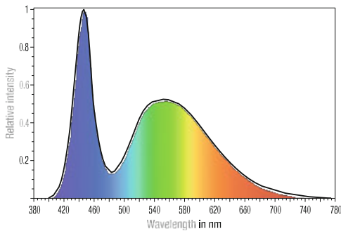
相対分光分布
