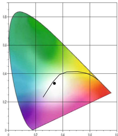
色度座標 X,Y CIE 1931
